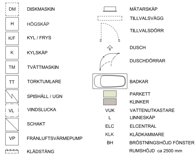
0 1 2 3 4 5 m SKALA 1:100
