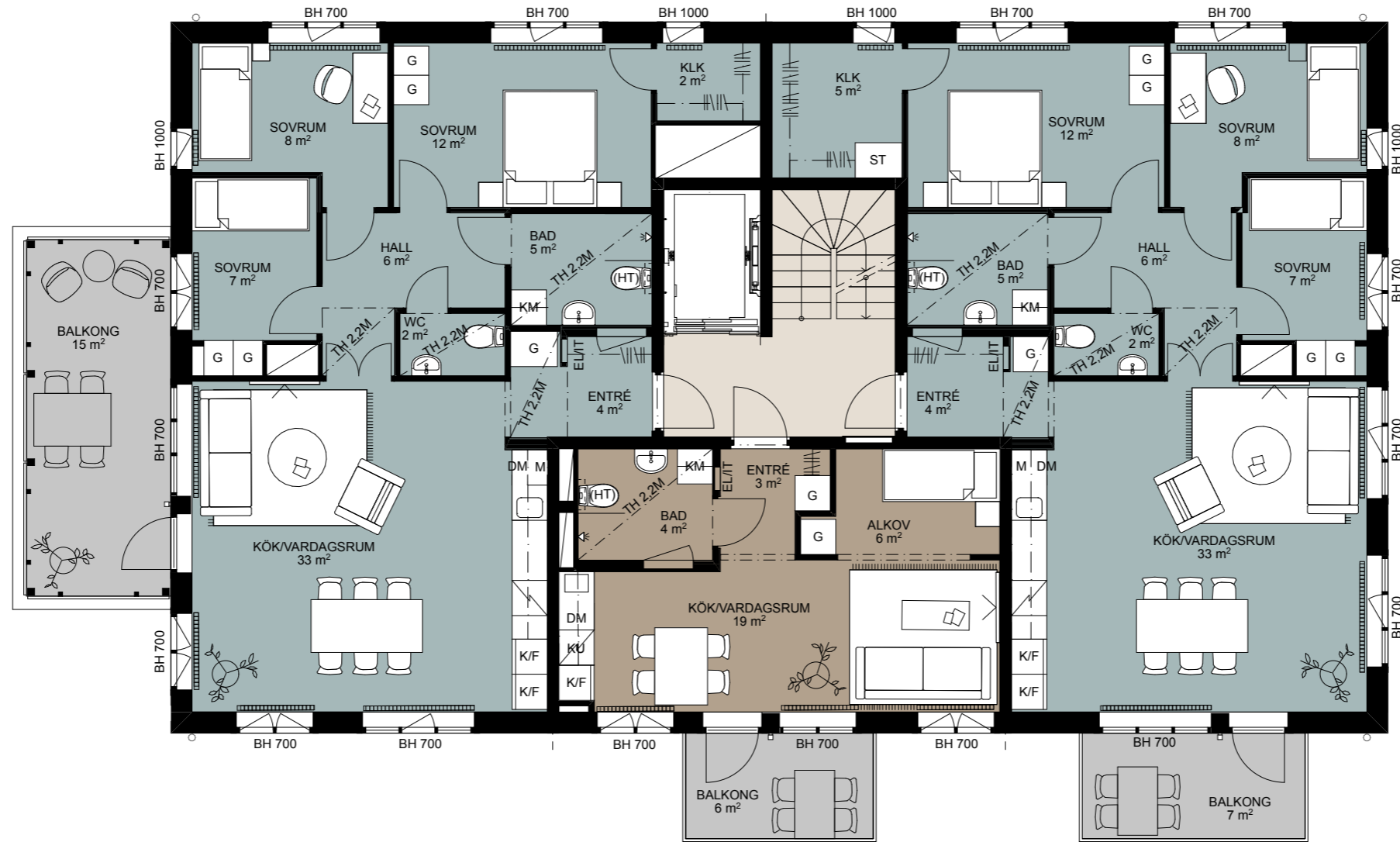
LÄGENHET 3-1102 1 rok, ca 32,8 m 2
