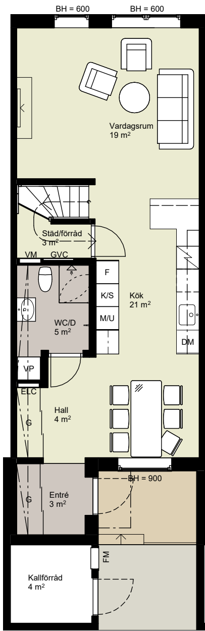
ENTRÉPLAN
