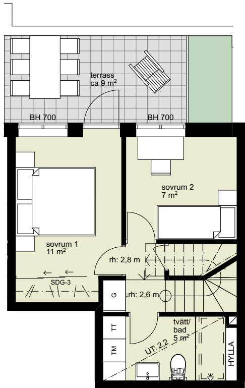
SUTERRÄNGPLAN
